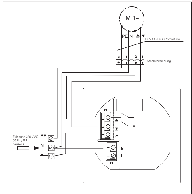
Abb. 6 Anschlussplan
