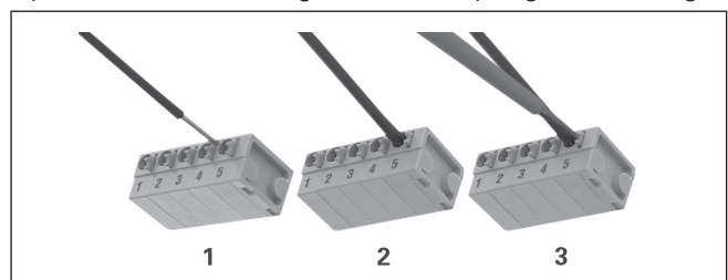
Abb. 2 Anschließen und Lösen der Leitungsverbindungen
