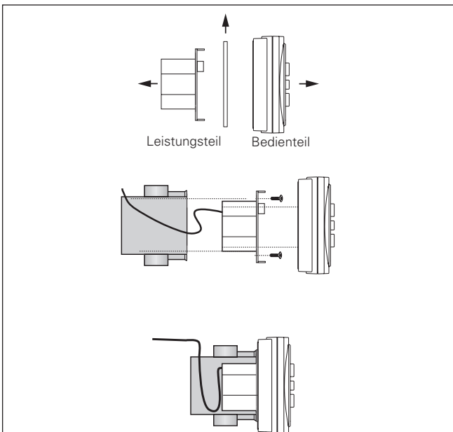
Abb. 4 Montage
