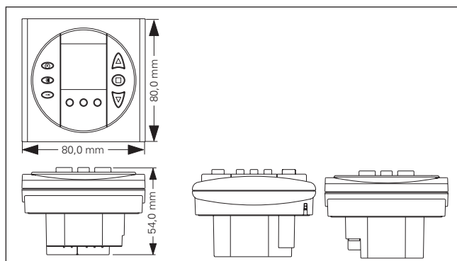
Abb. 8: Abmessungen
